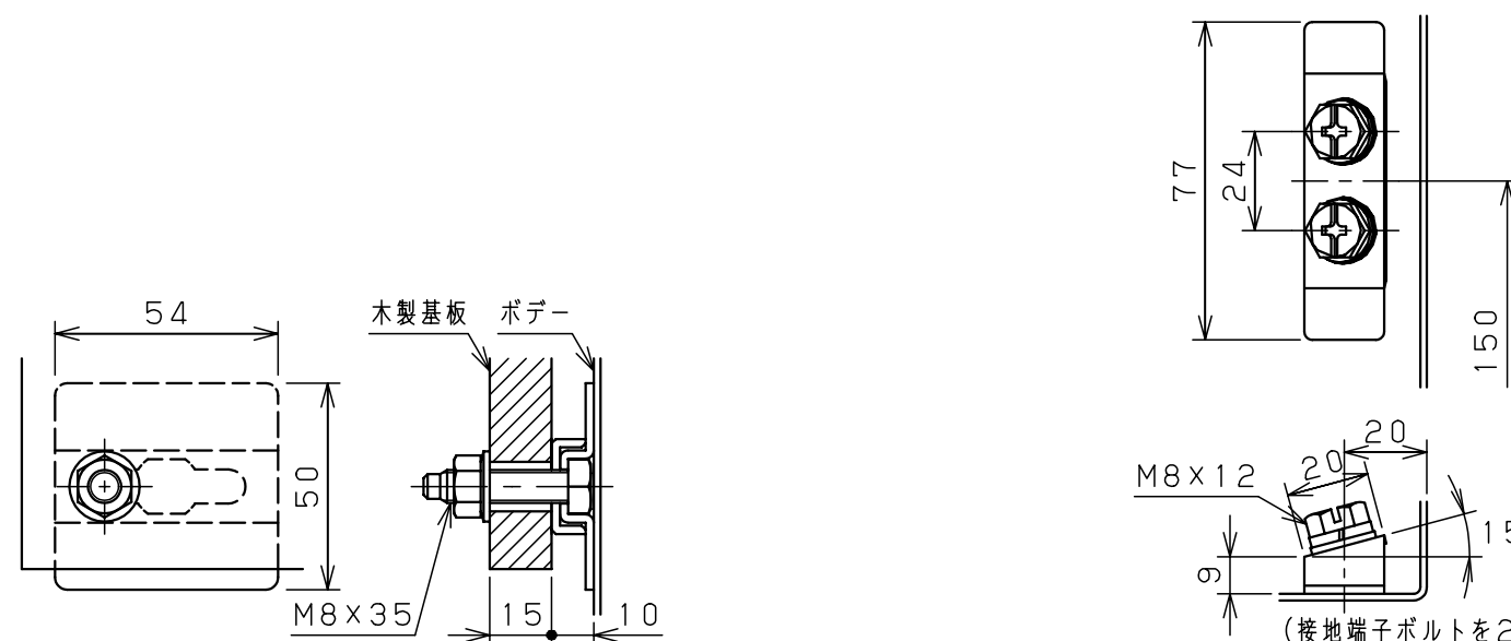
基板取付部詳細 (1 : 2)
