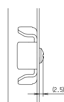
D部詳細 (1:1)
