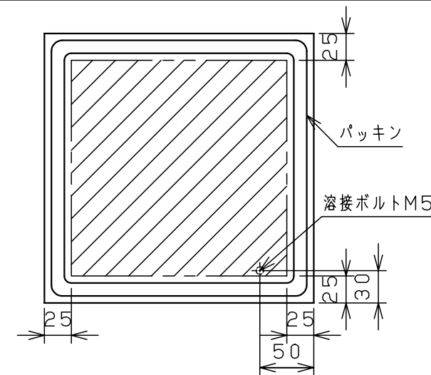
扉 機器取付有効図
