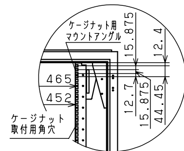
マウントアングル詳細図 (1:15)
