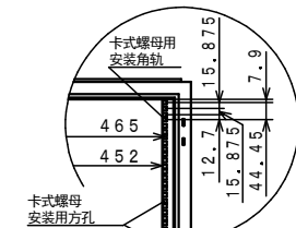
安装角轨局部放大图 (1:15)
