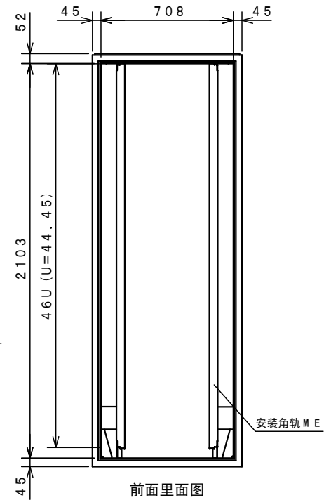
前面里面图
