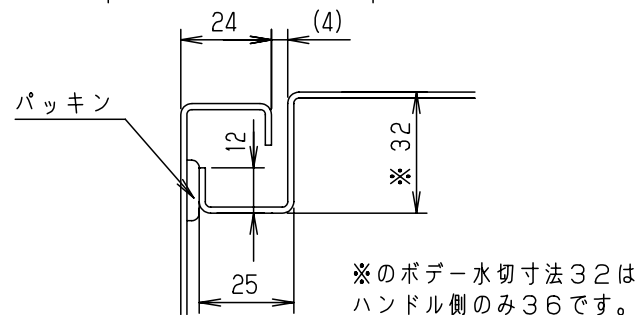
A部断面詳細（1：2）
