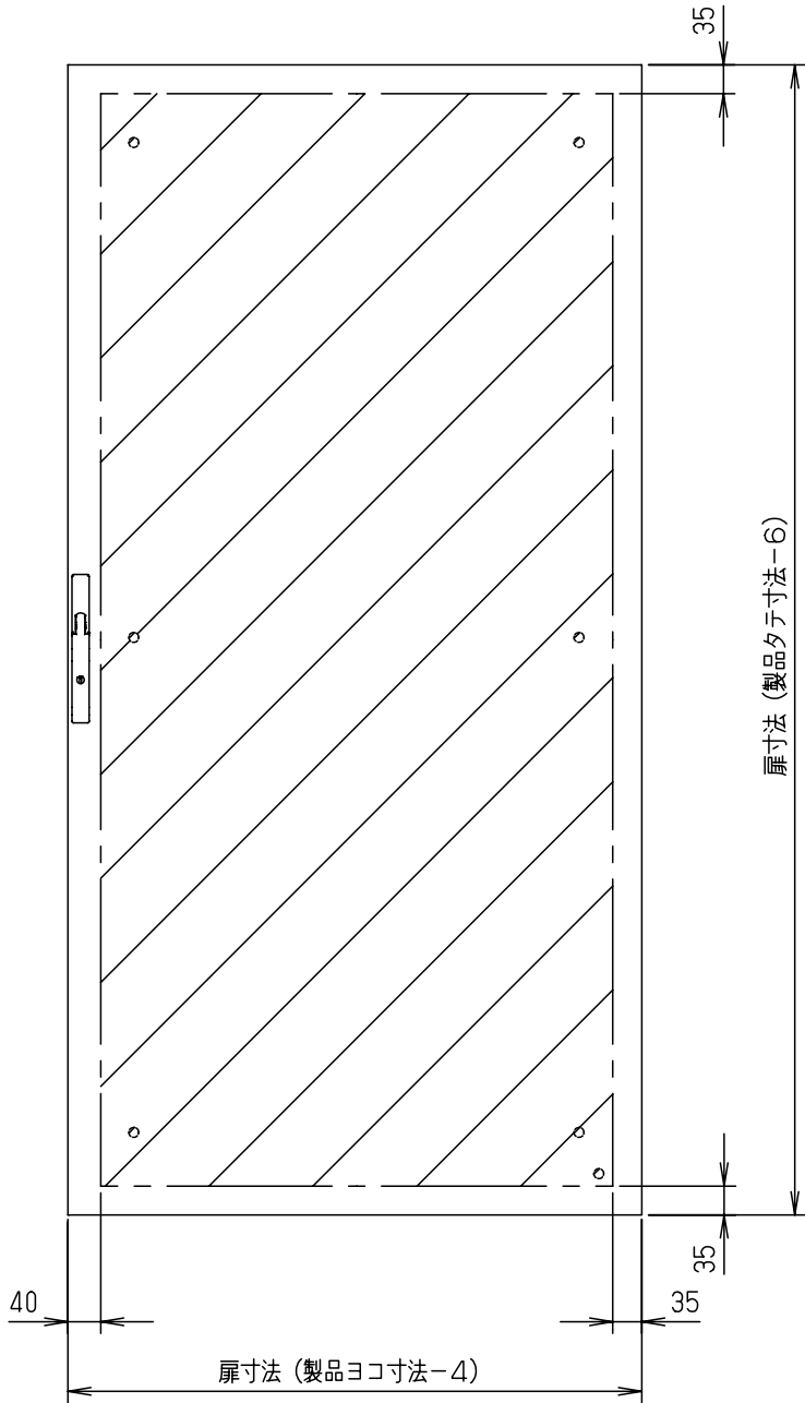
扉機器取付有効図
