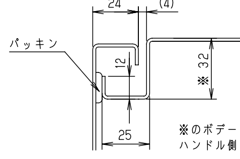
A部断面詳細（1：2）
