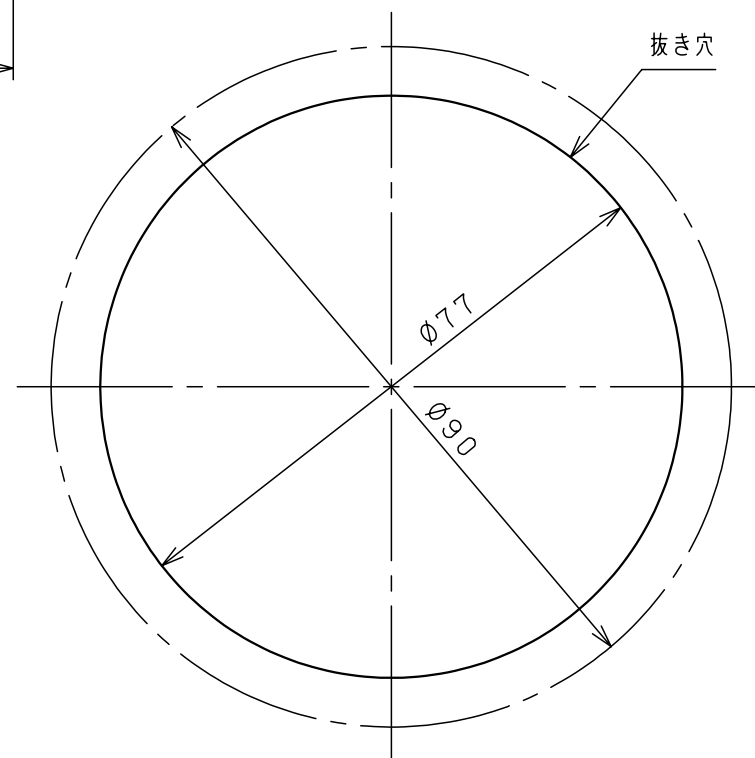
取付寸法図
