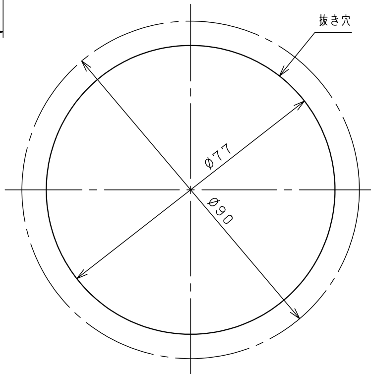
取付寸法図
