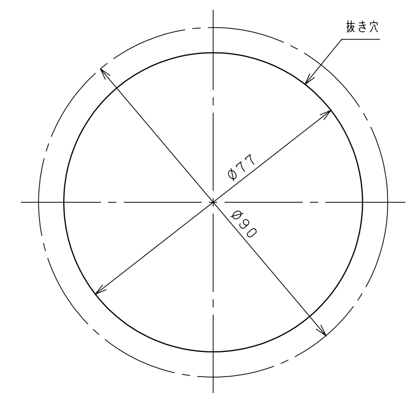
取付寸法図 一点鎖線は本器外形を示します。
