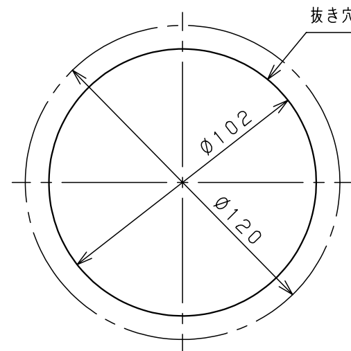
取付寸法図 (1:2)
