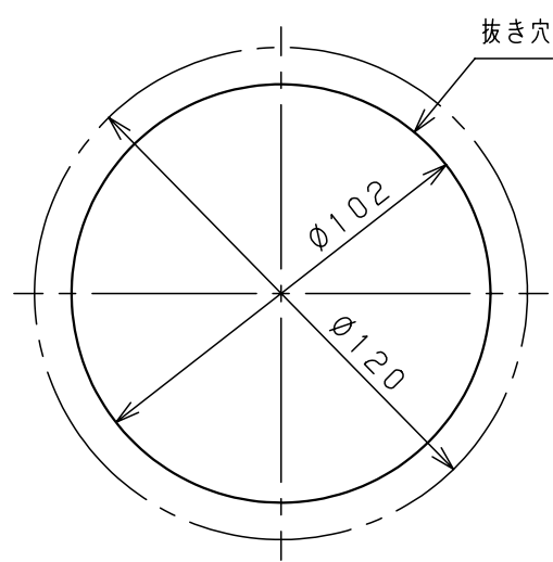
取付寸法図 (1:2)
