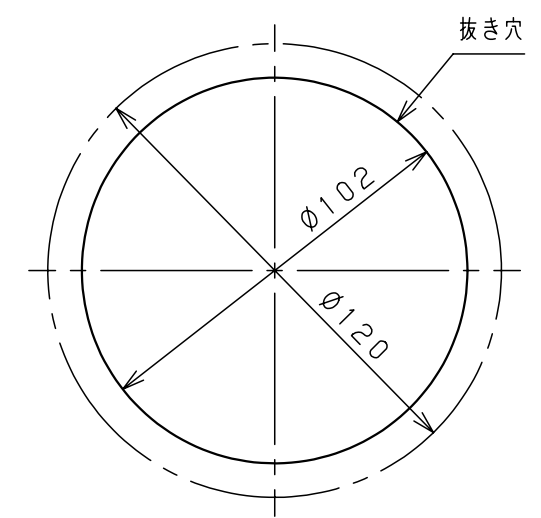
取付寸法図 (1:2) 一点鎖線は本器外形を示します。
