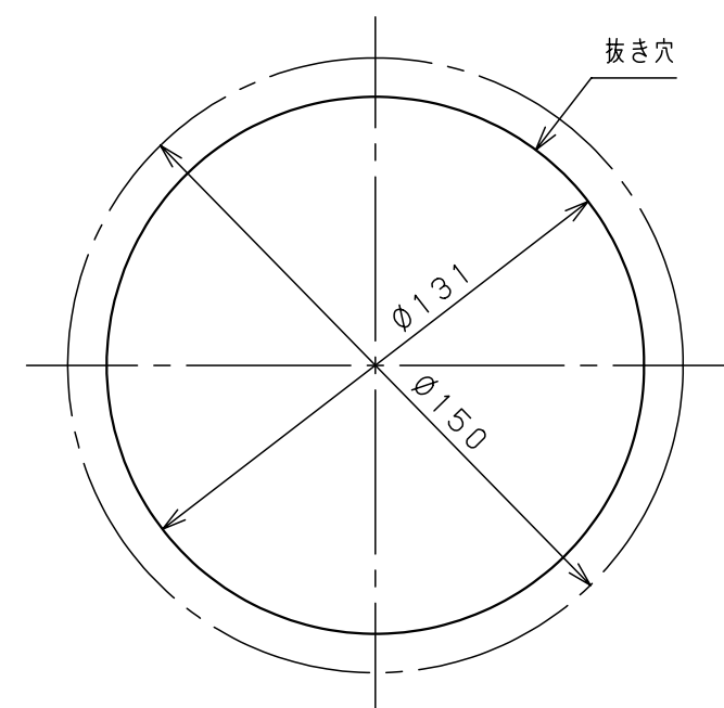
取付寸法図
