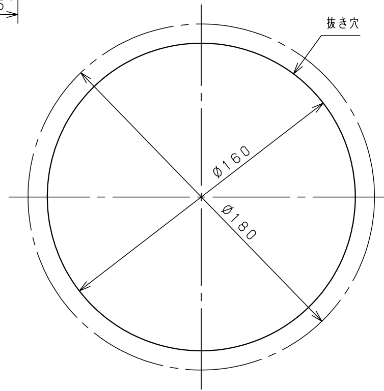
取付寸法図
