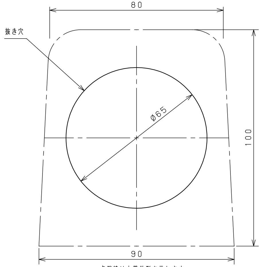
取付寸法図
