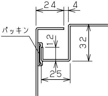
A部断面詳細 (1:2)
