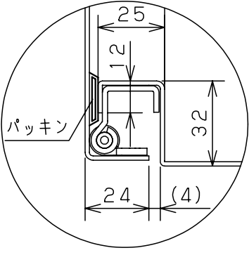
B部断面詳細 (1:2)
