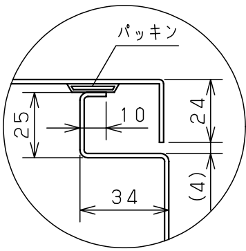
A部断面詳細 (1:2)
