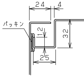
A部断面詳細 (1:2)
