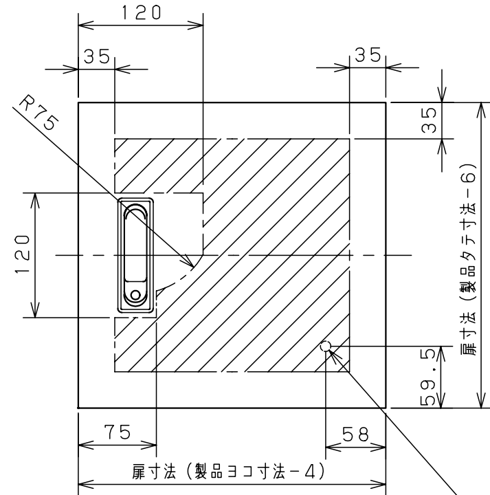
溶接ナットM5 (扉裏面、アース用)
