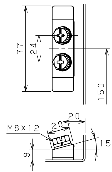
B部接地端子詳細 (1:2) (国土交通省仕様)
