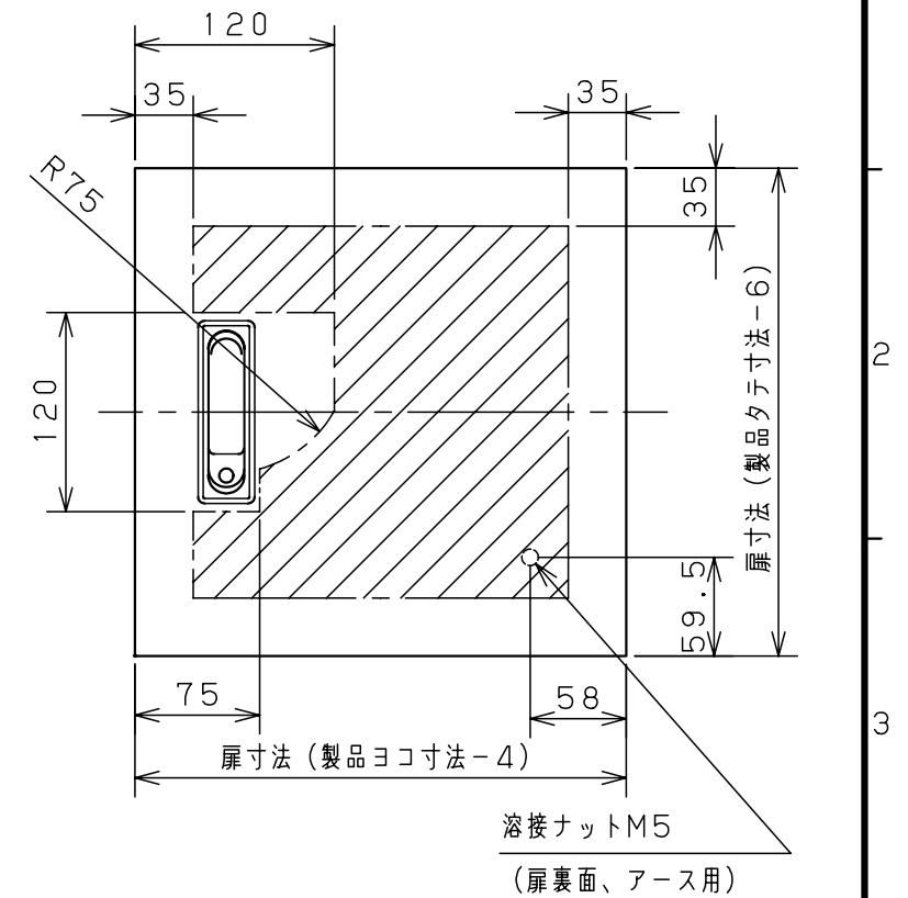
扉機器取付有効図
