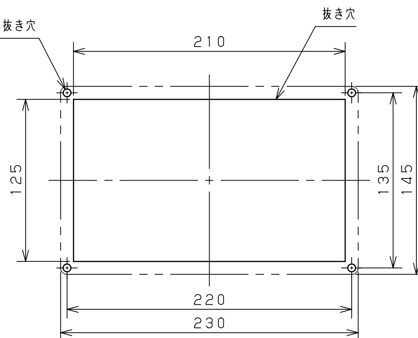
取付寸法図
