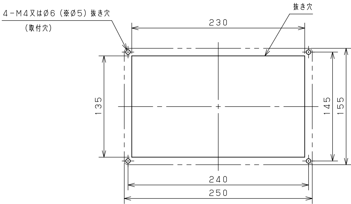
取付寸法図
