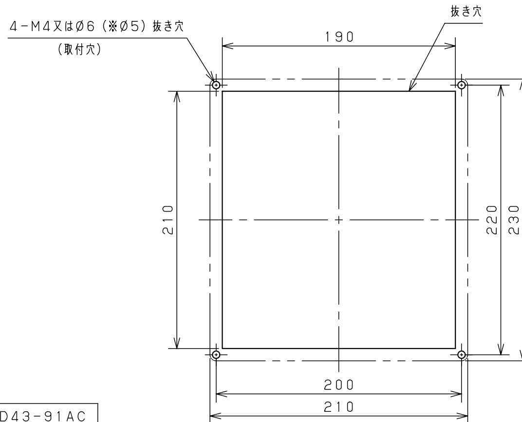
取付寸法図
