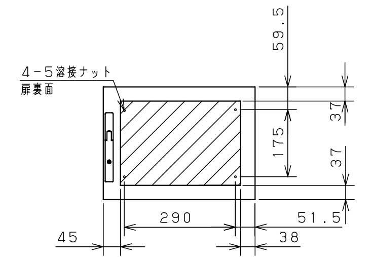
扉 機器取付有効図
