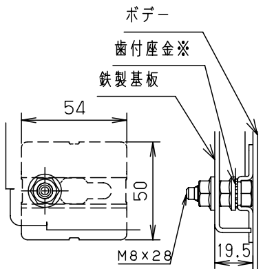
基板取付部詳細 (1:2)
