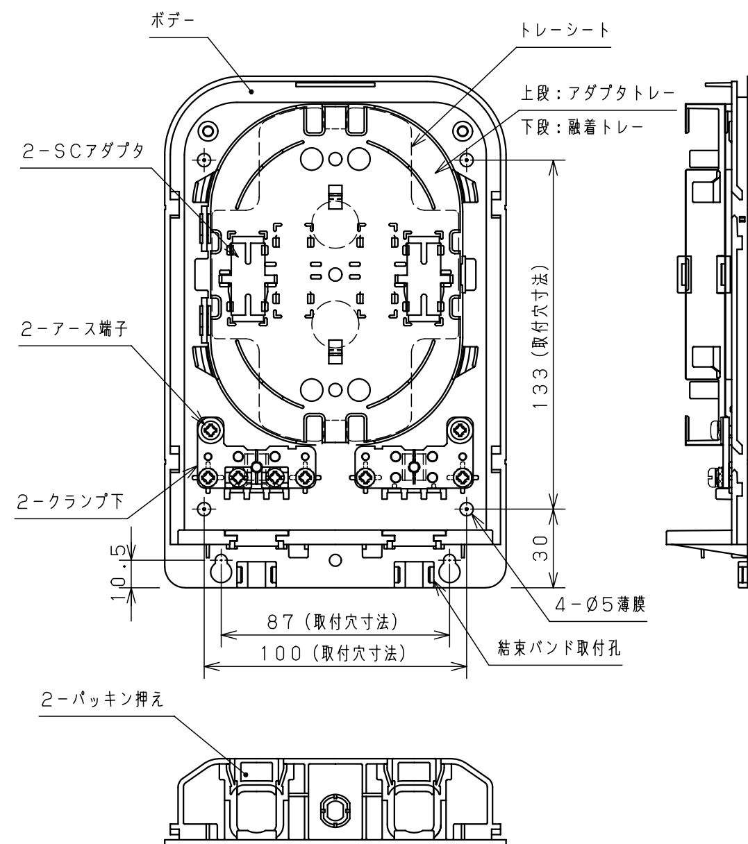
内部詳細図
