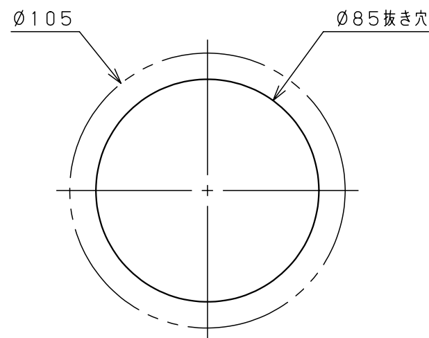
取付寸法図
