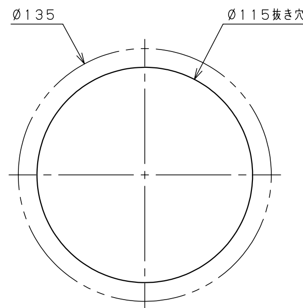
取付寸法図
