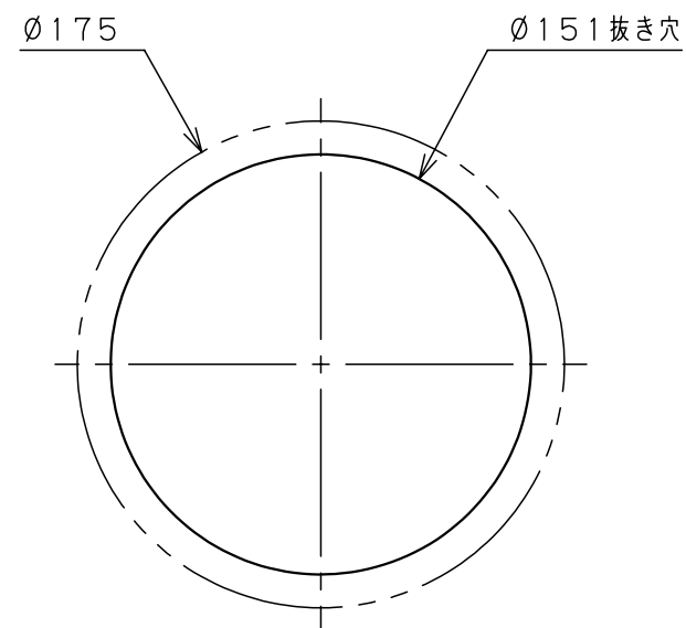
取付寸法図
